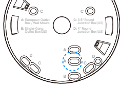
A: European Outlet Box
